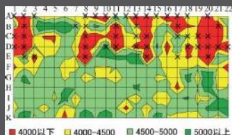
後半機械インピーダンス値の等価線図
