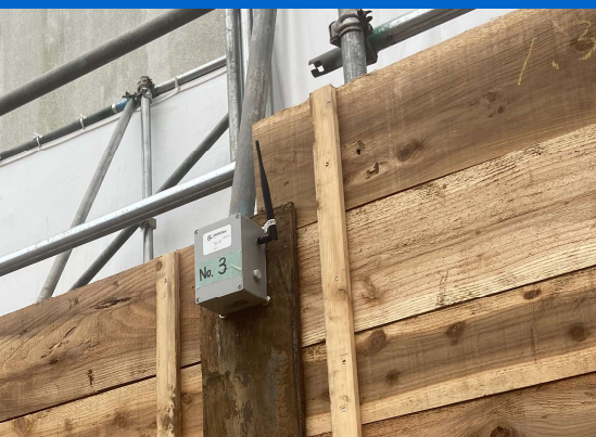
土留め壁・矢板の変位計測
