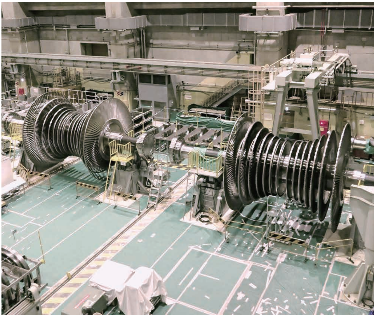
島根原子力発電所2号機 蒸気タービンローター(中国電力(株)提供)
